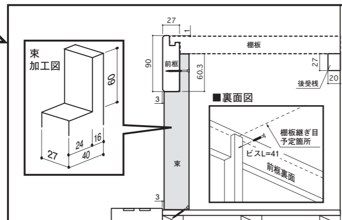
図2.束取り付け断面図
