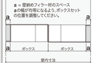
【上面図】
