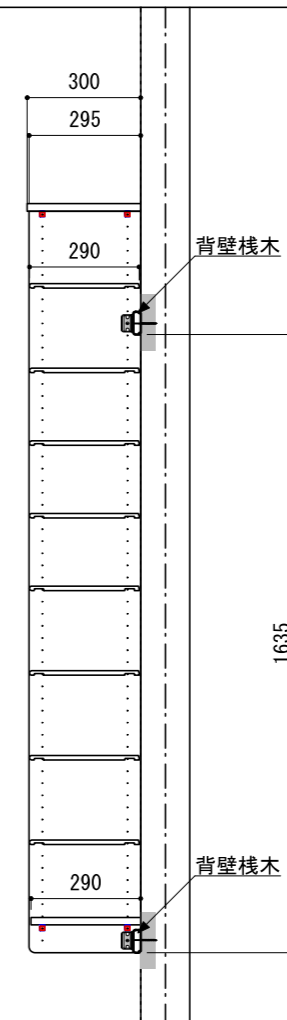
A-A' 断面
