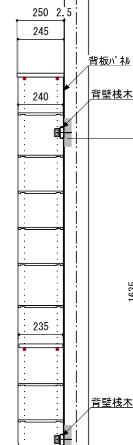
A-A' 断面
