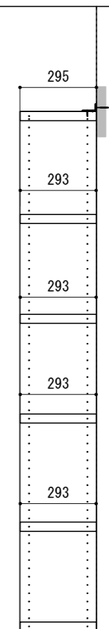
A-A' 断面
