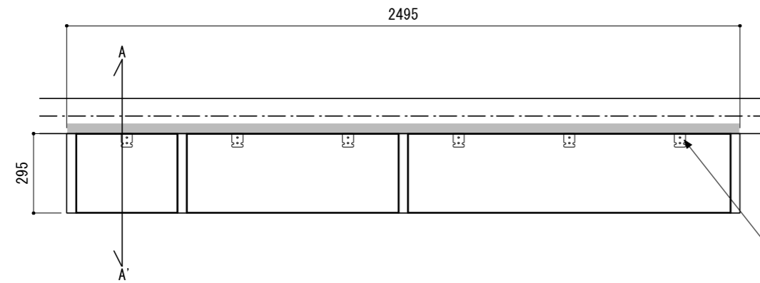
背壁固定用ブラケット+カバーキャップ(同梱)
