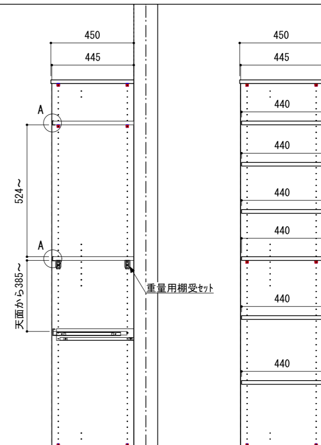
A-A' 断面
