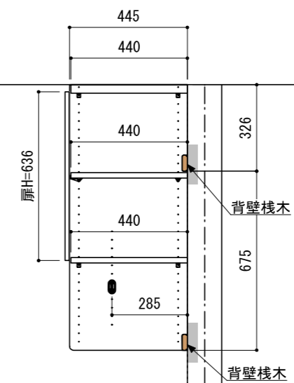
A-A' 断面
