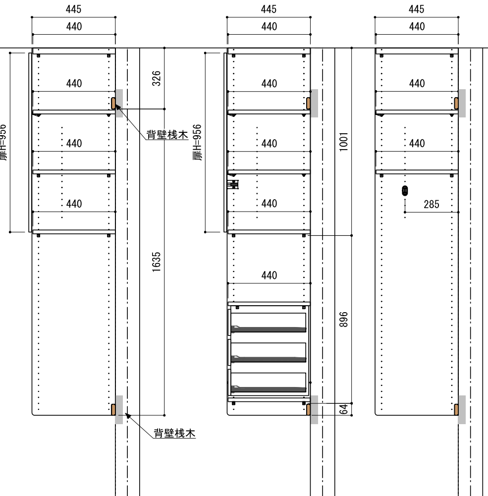
A-A' 断面
