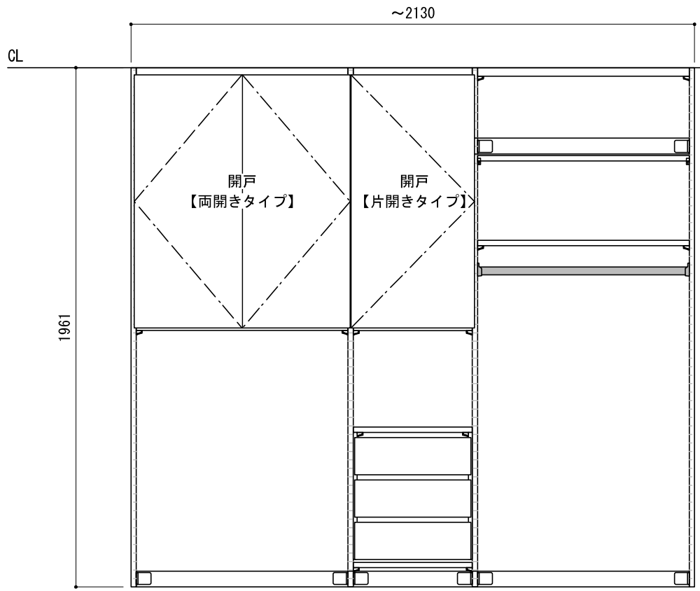
正面図（外観）
