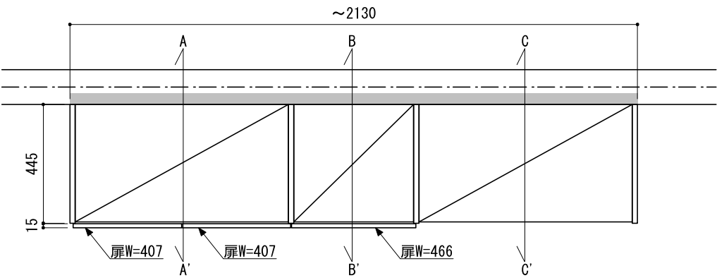
正面図（外観）
