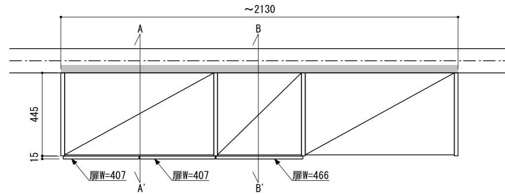
正面図（外観）
