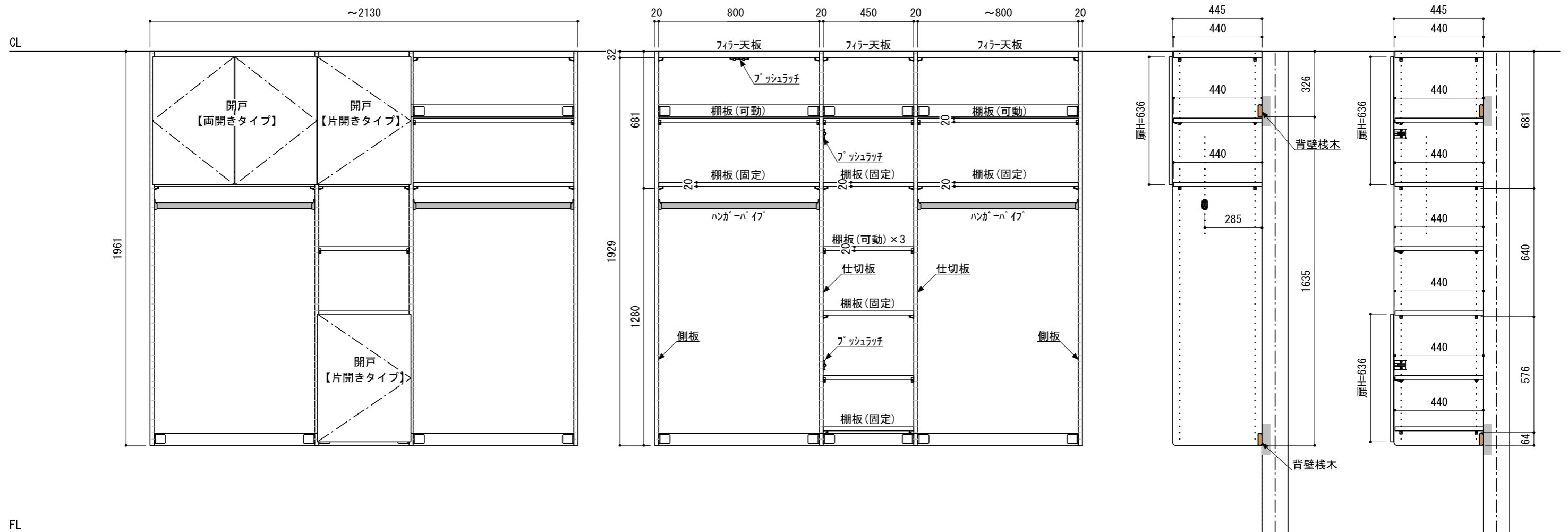
A-A' 断面
