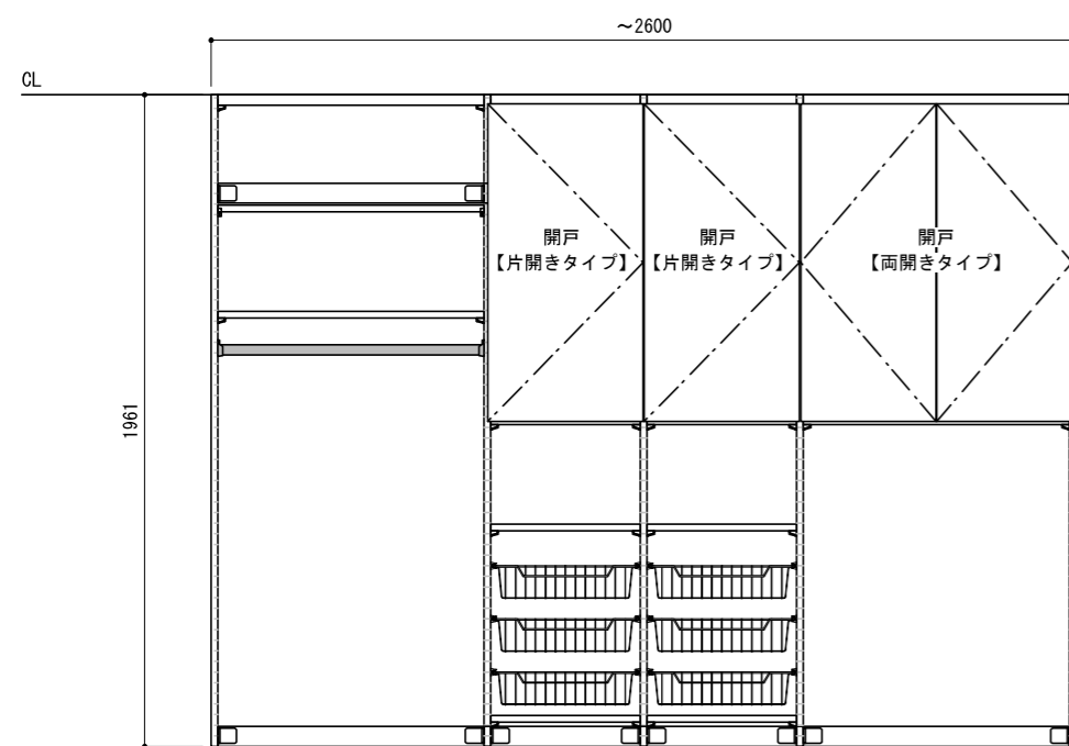
正面図（外観）
