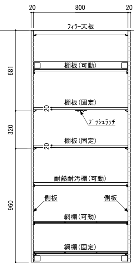
正面図（扉内部）
