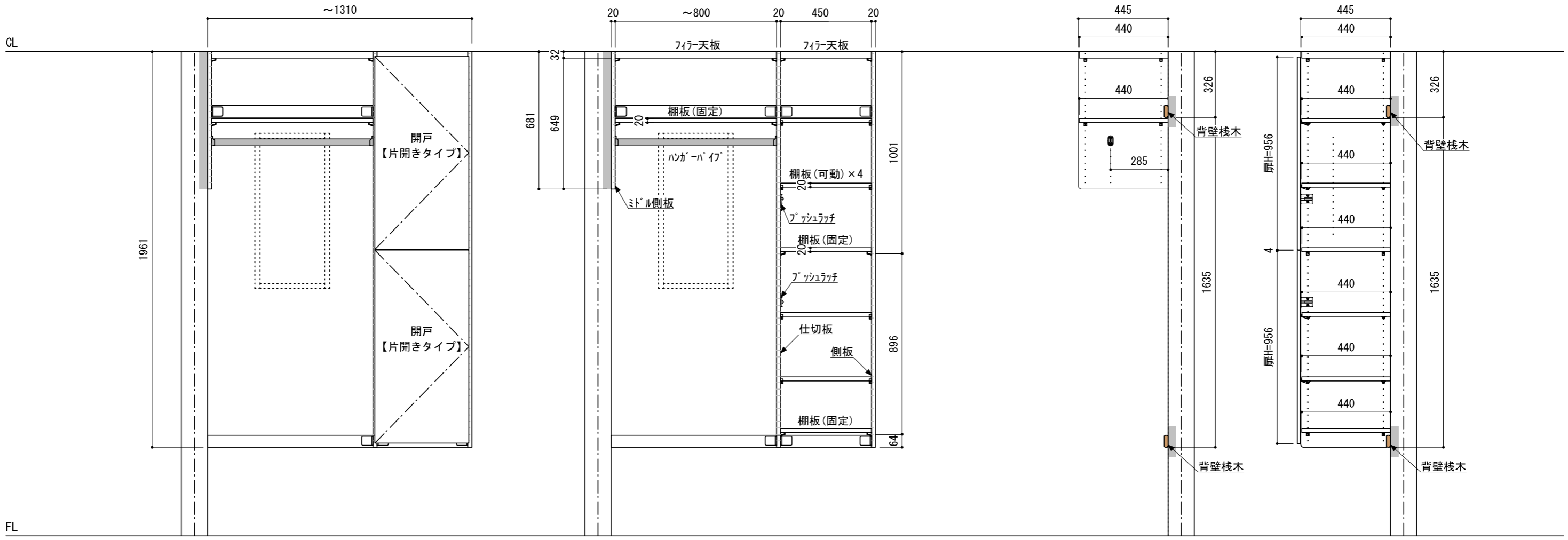
正面図（外観）
