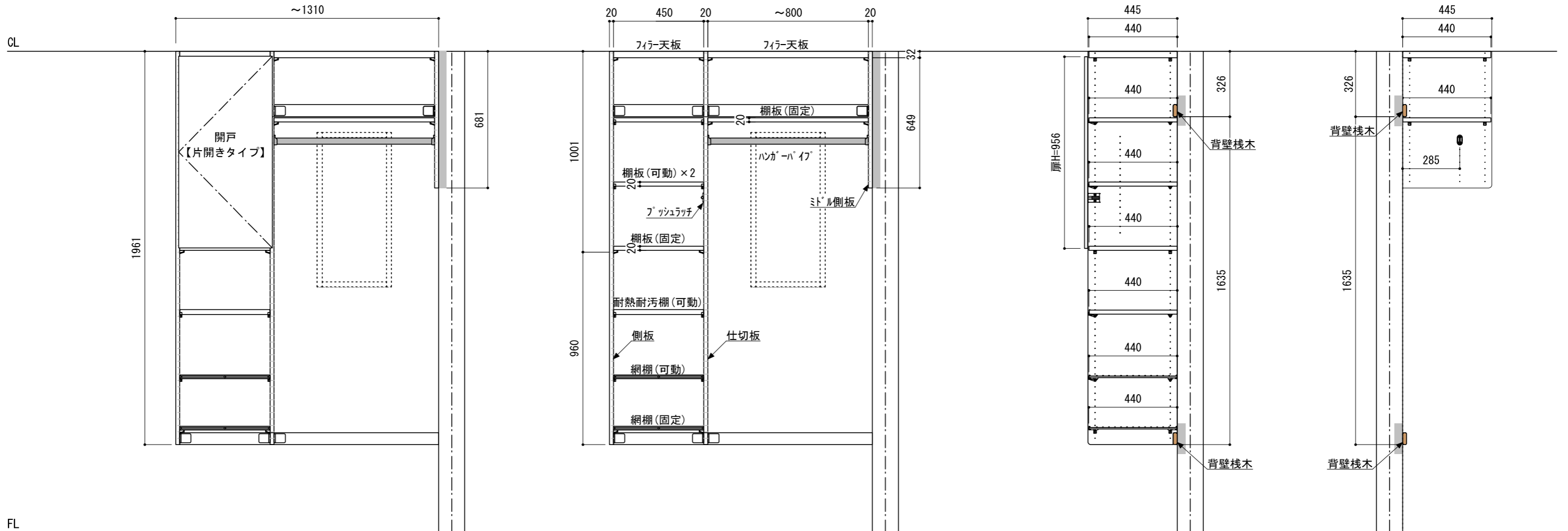
正面図（外観）
