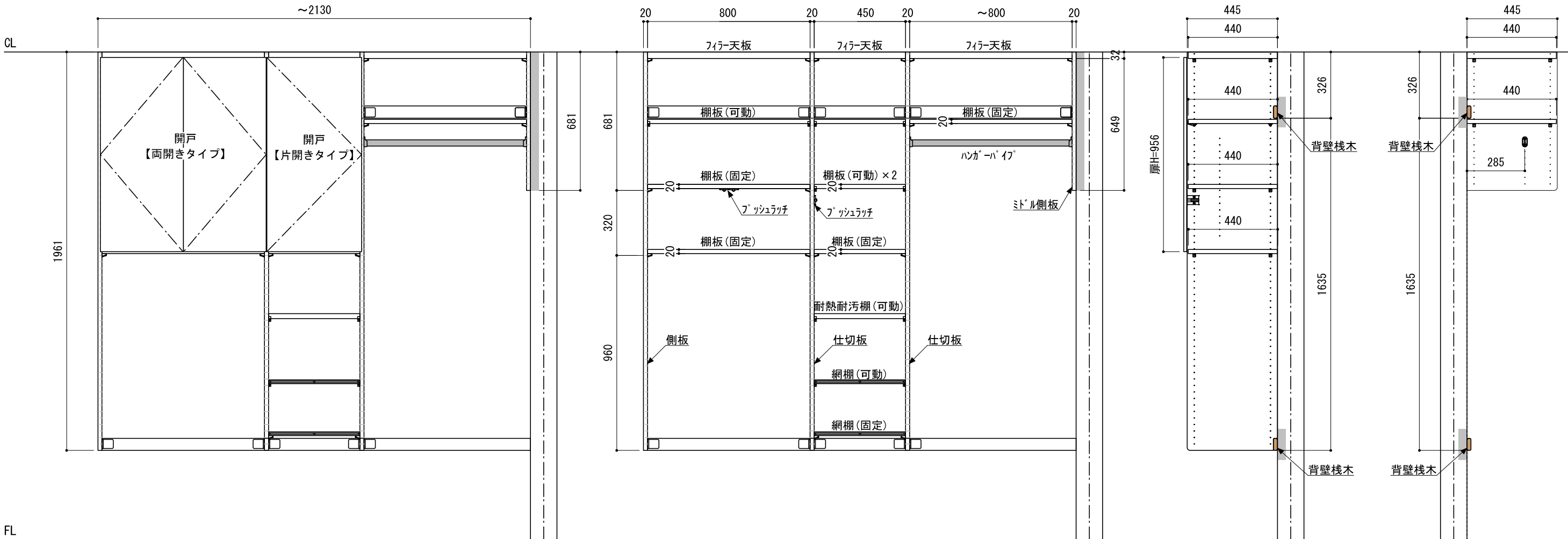
正面図（外観）
