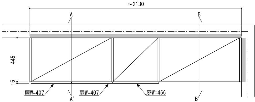
正面図（外観）
