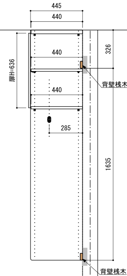
A-A' 断面
