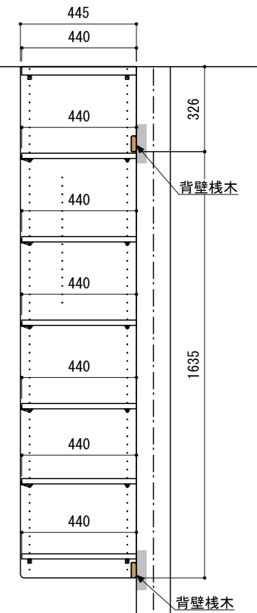
B-B' 断面
