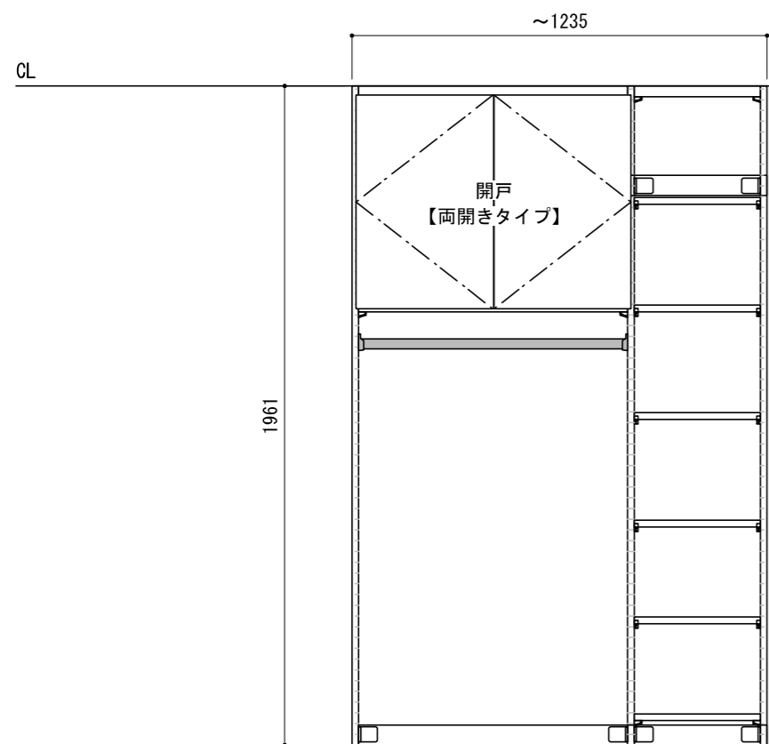
正面図（外観）
