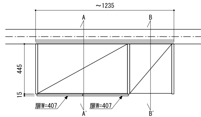
正面図（外観）
