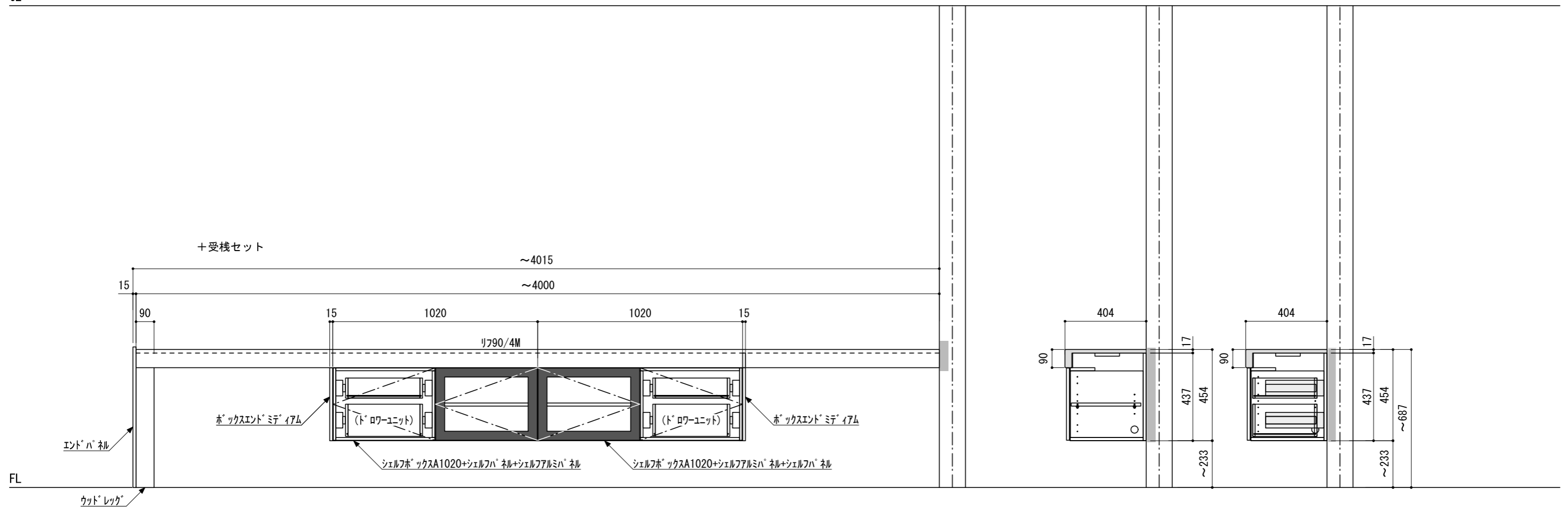
A-A' 断面
