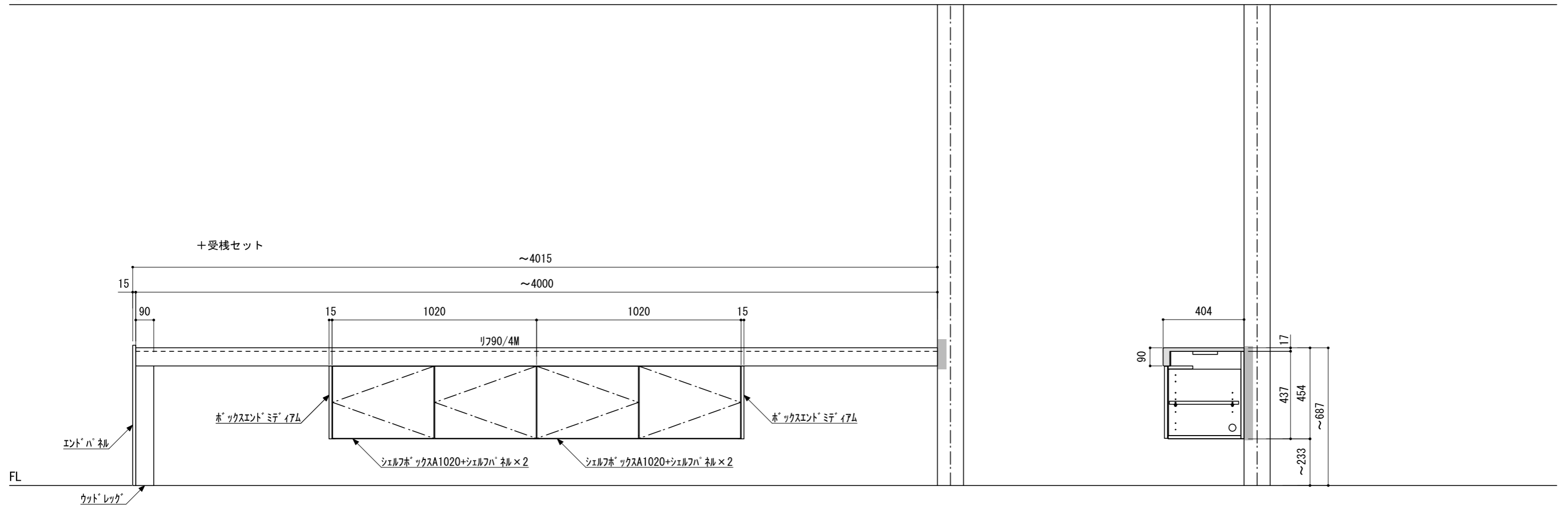
A-A' 断面
