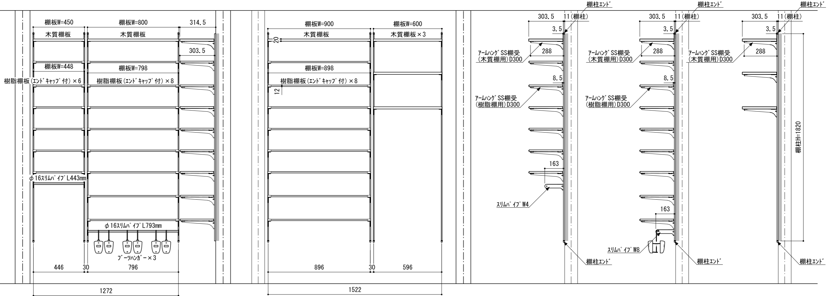
A立面
