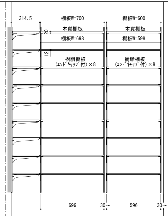
B 立面
