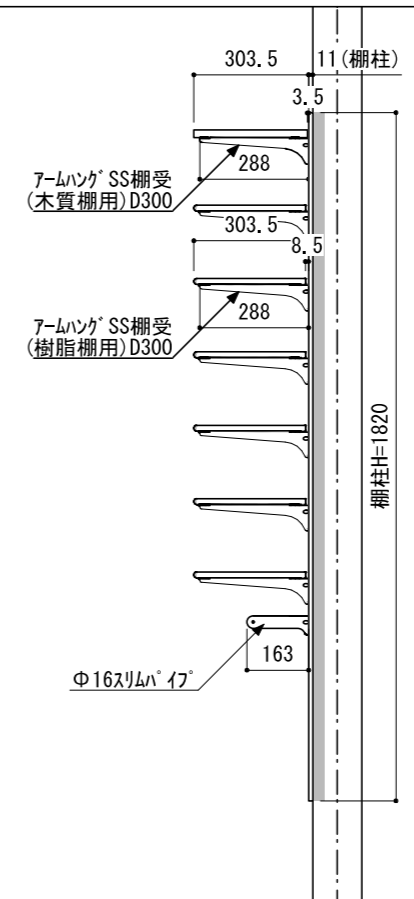
A-A' 断面
