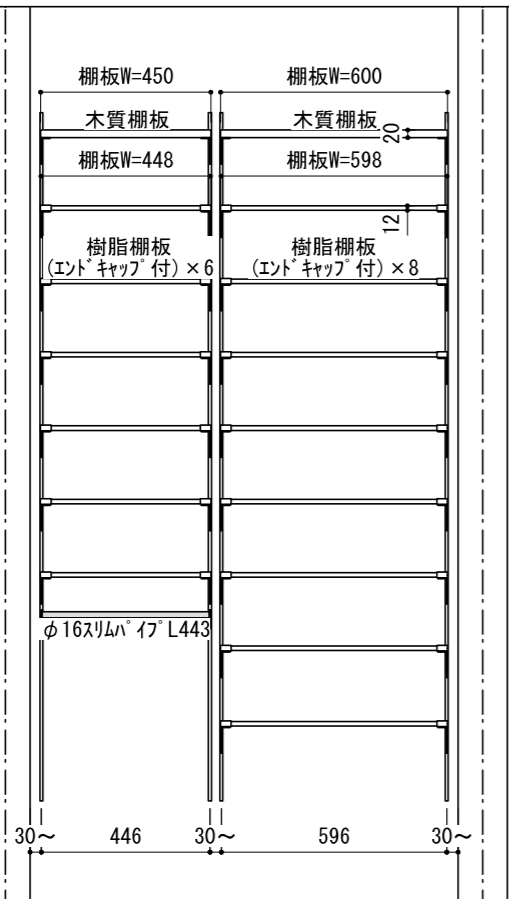
A 立面
