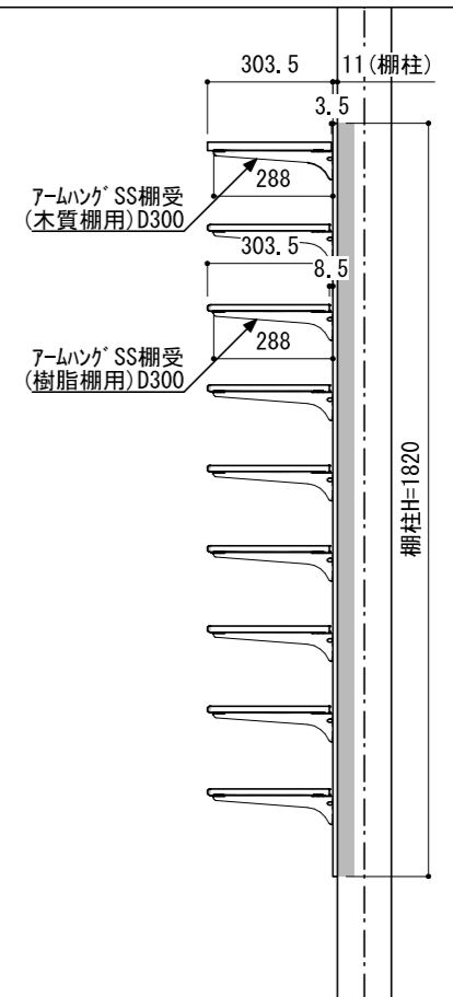
B-B' 断面
