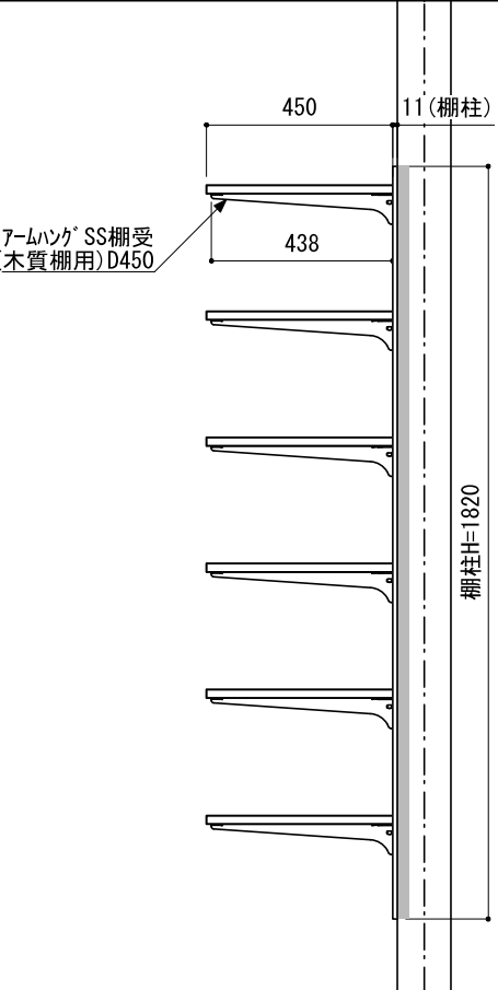
A-A' 断面
