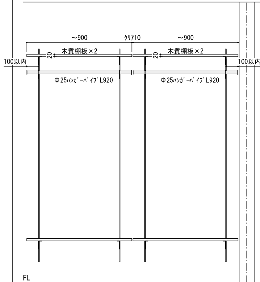
A 立面
