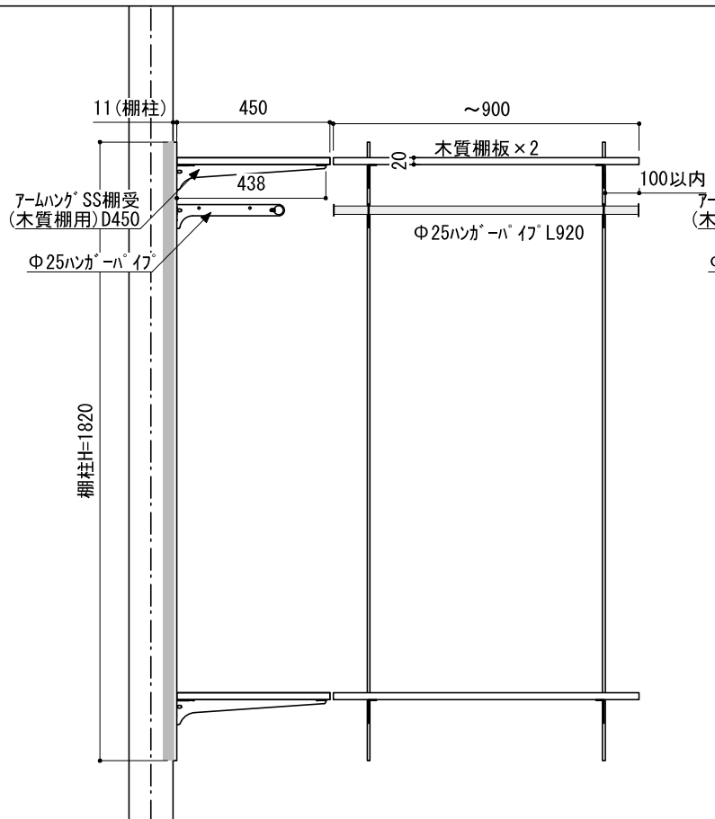
C 立面
