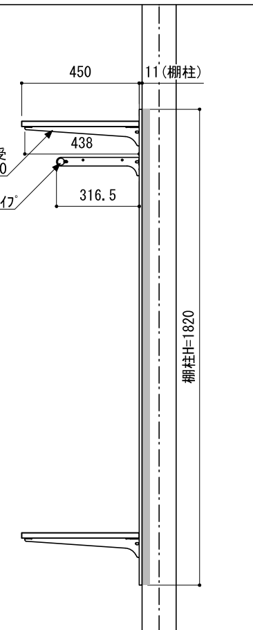
A-A' 断面
