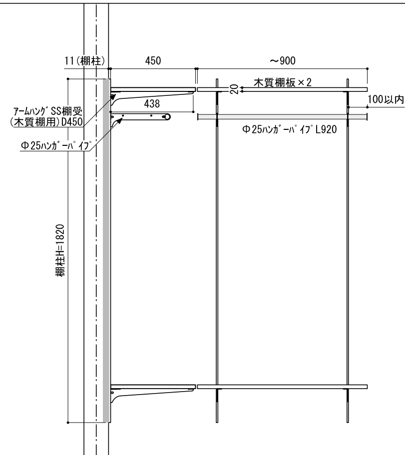
B 立面
