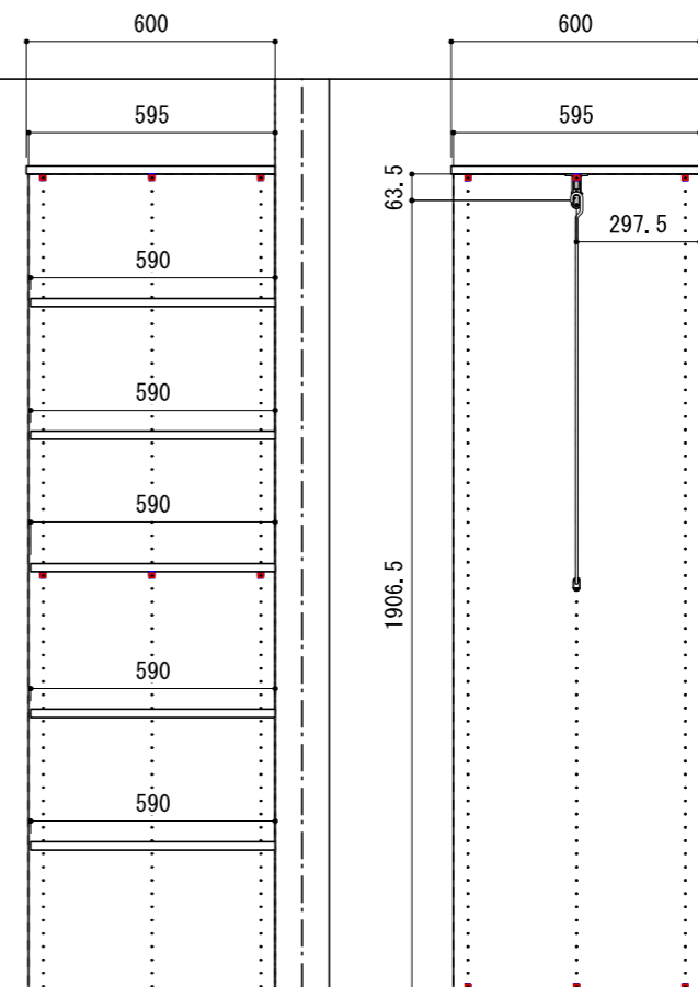
A-A' 断面
