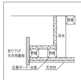
「折り下げ天井用幕板」使用例
