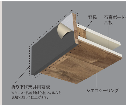
「折り下げ天井用幕板」使用例
