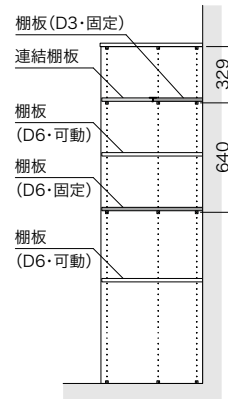
[B-B'断面図]
