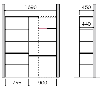
奥行450
