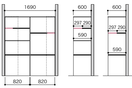
奥行600
