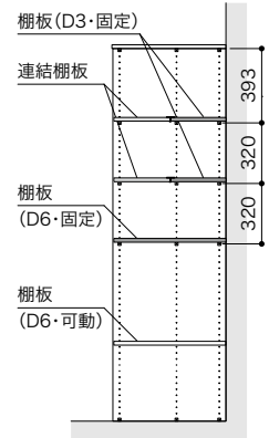
[C-C'断面図]
