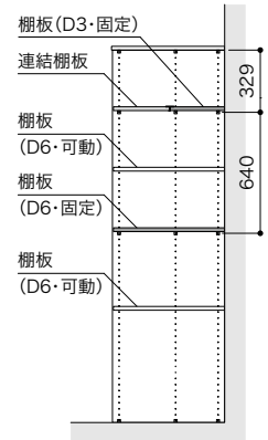
[C-C'断面図]
