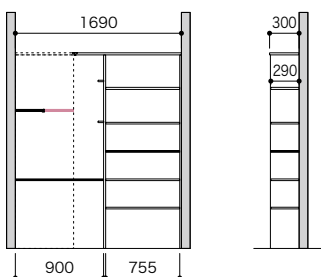
奥行300
