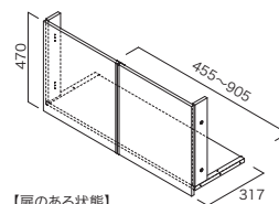
【扉のある状態】
