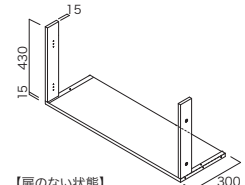
【扉のない状態】
