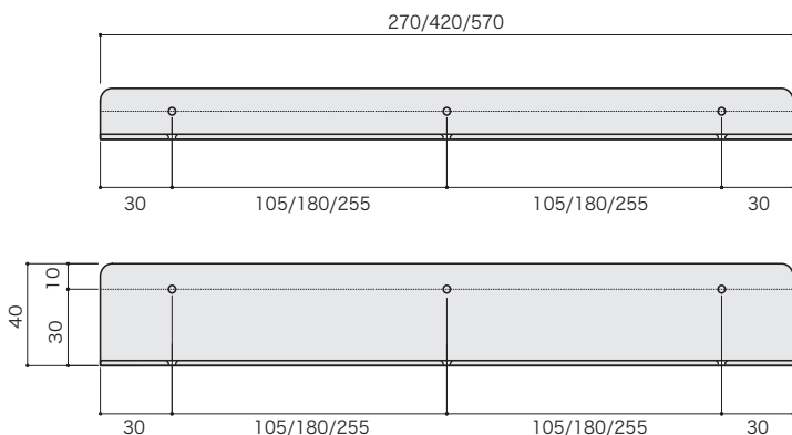
[ 寸法図 ]
