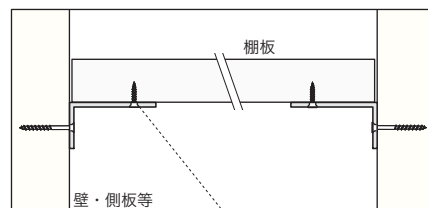
[ 納まり図 ]
