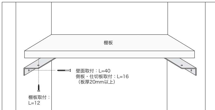
[ 推奨取付図 ]
