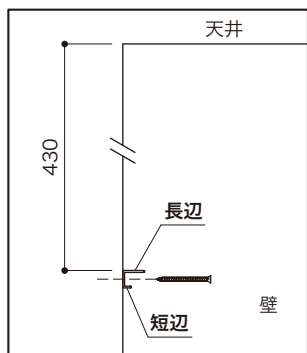
〔底板レールの取り付け位置〕
