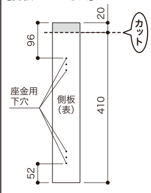
【側板カット寸法】
