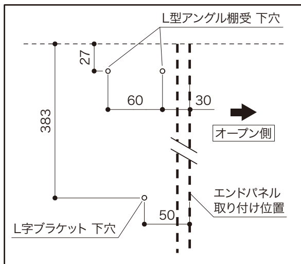
【L型アングル棚受・L字ブラケット 下穴位置】
