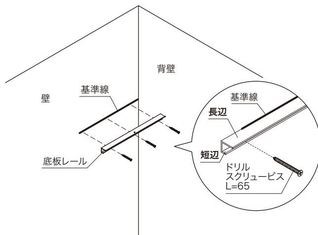
〔底板レールの取り付け位置〕
