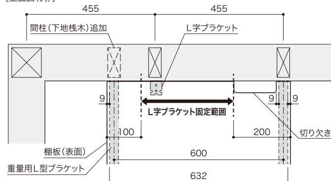
【上面図(例)】
