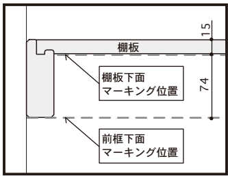
マーキング位置 (断面図)
