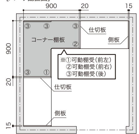
[パーツ配置図]
