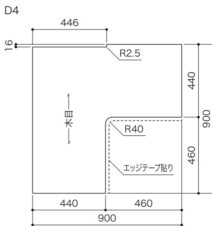
[パーツ配置図]
