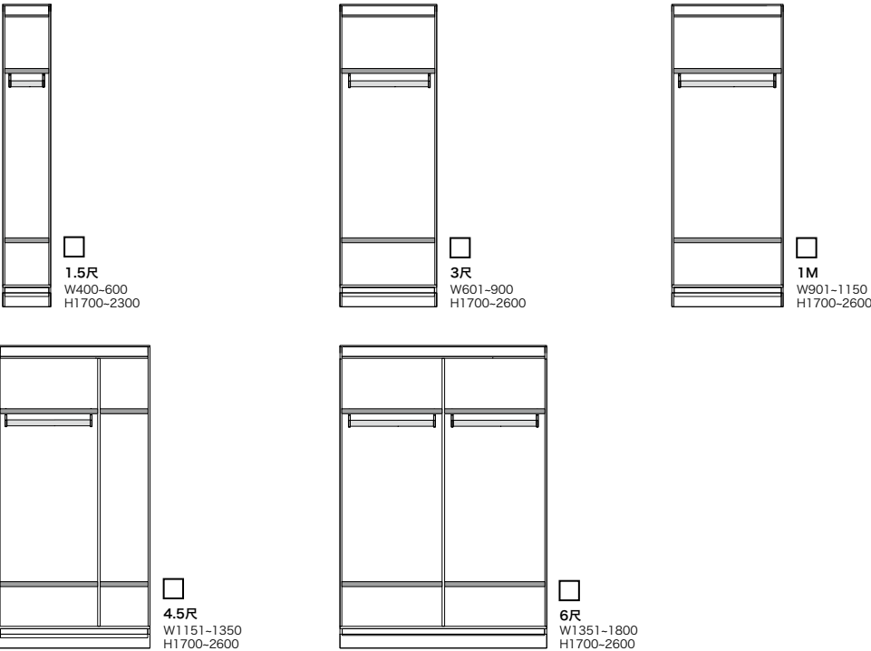
図は特寸サイズのボックス内部基本セット内容・設置位置
