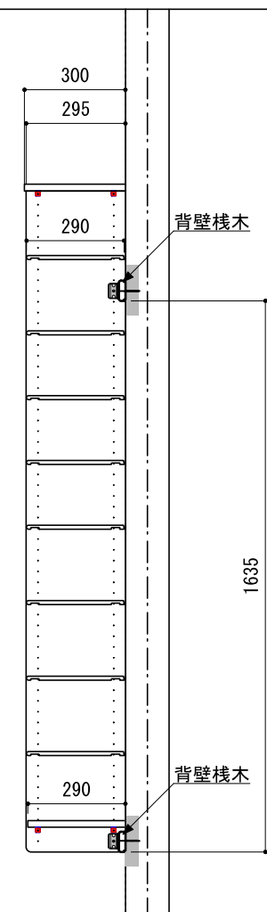
A-A' 断面
