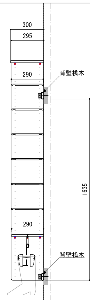
A-A' 断面
