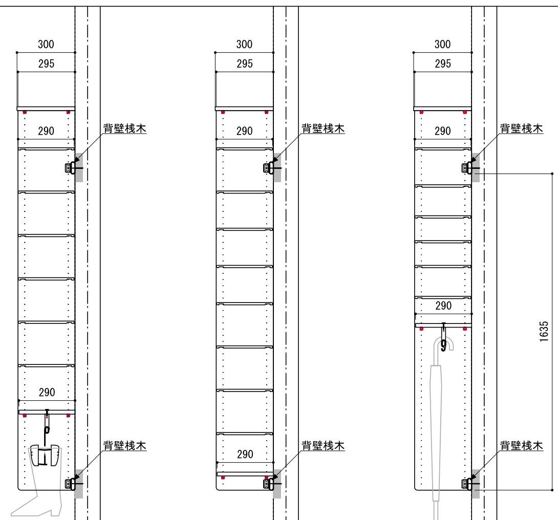
A-A' 断面
