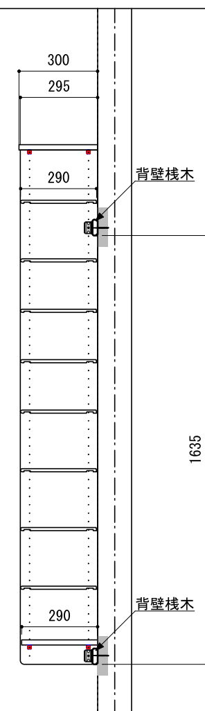
B-B' 断面
