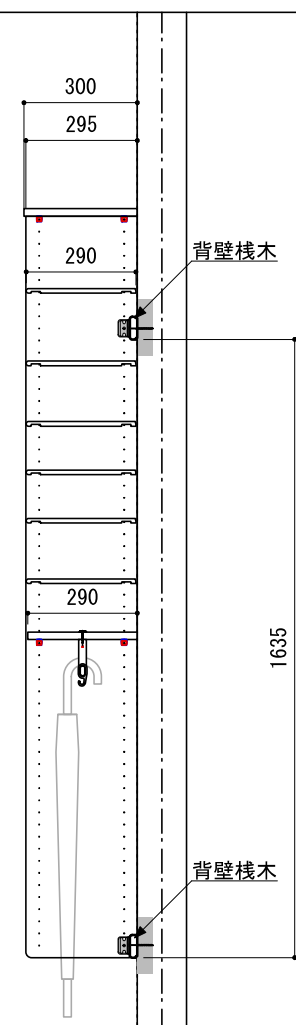
C-C' 断面
