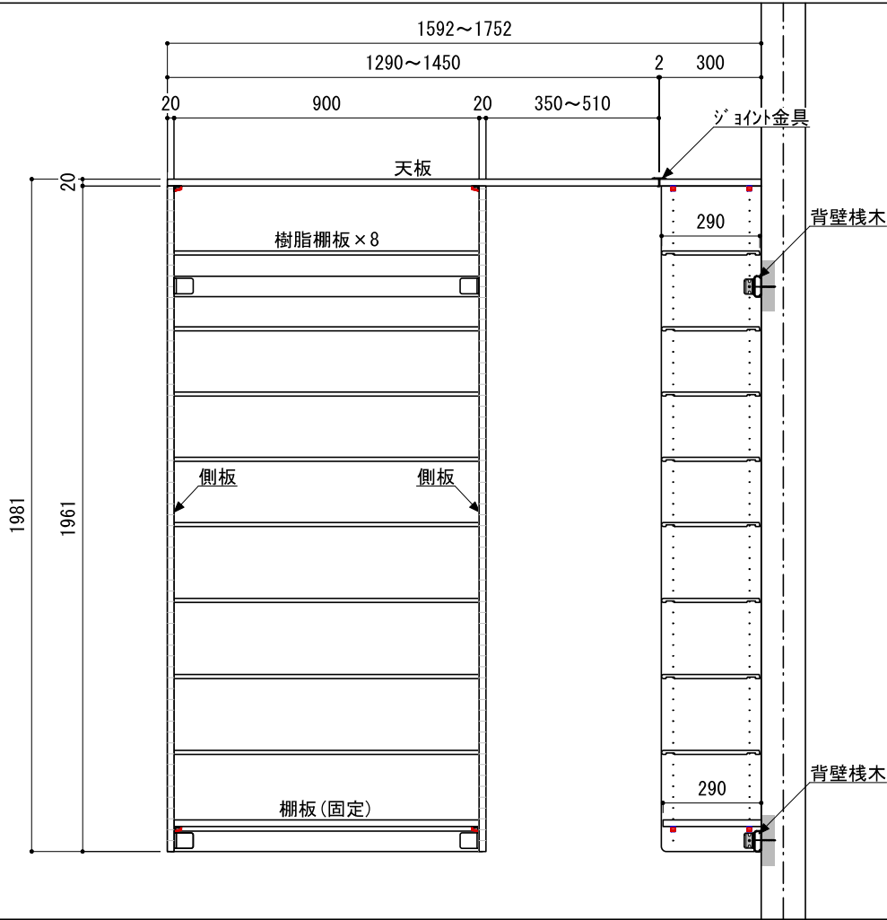
A 立面
