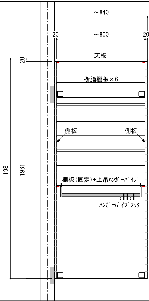
C立面
