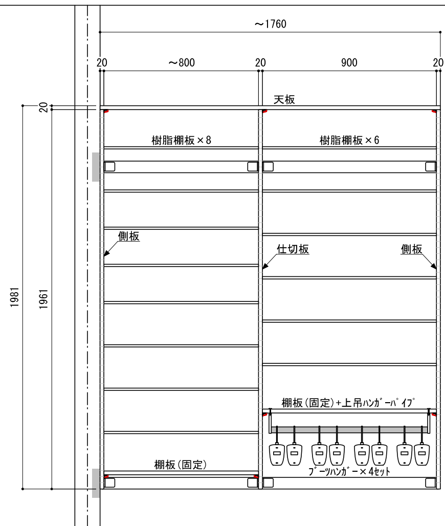
C立面
