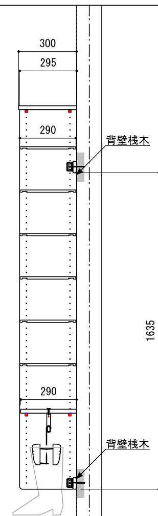
C-C' 断面
