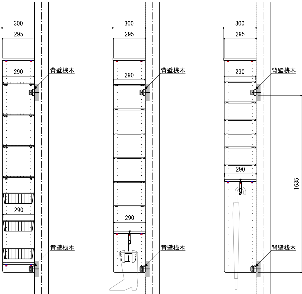
A-A' 断面
