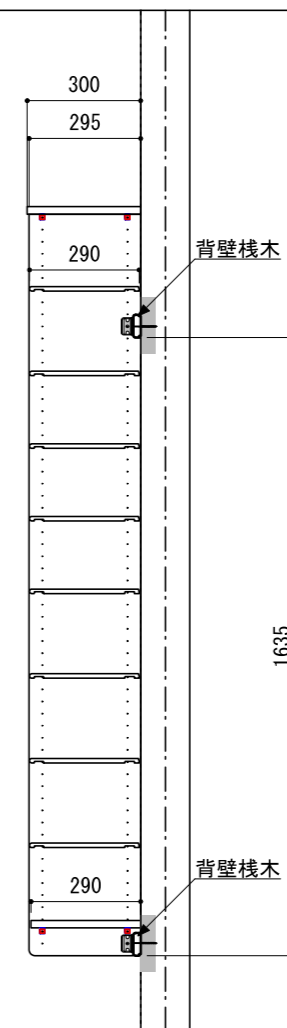
A-A' 断面
