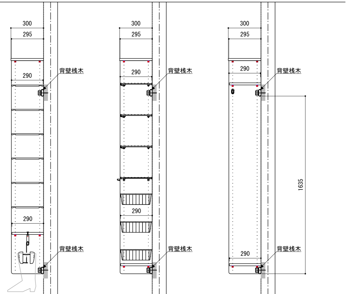
A-A' 断面
