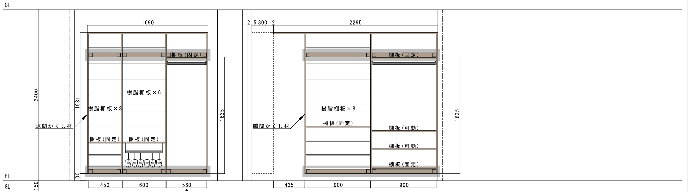
① 立面
