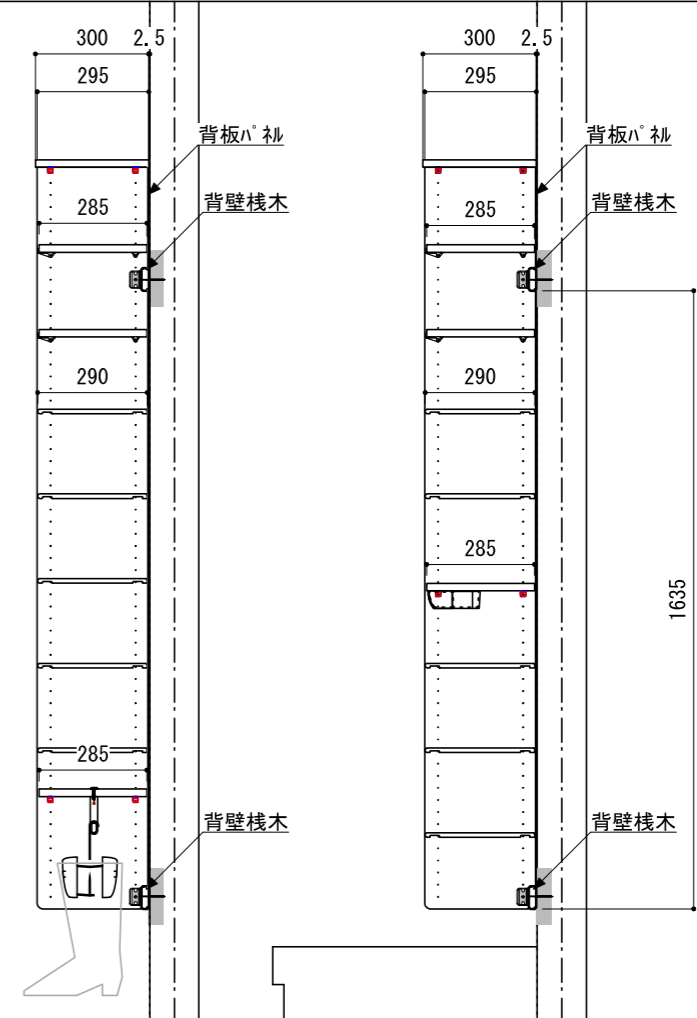
A-A' 断面
