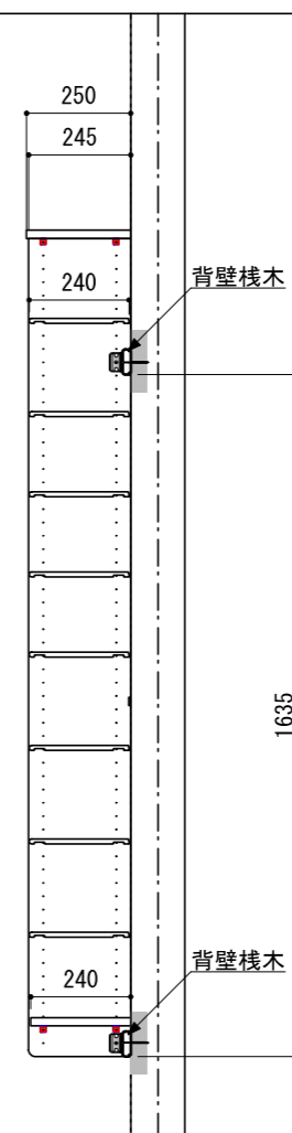
A-A' 断面
