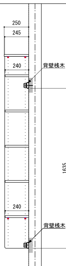
A-A' 断面
