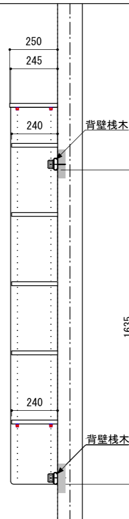
A-A' 断面
