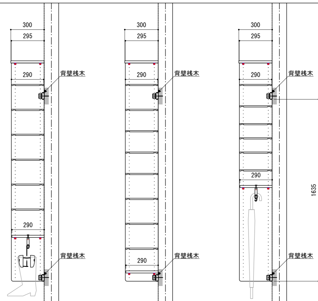
A-A' 断面
