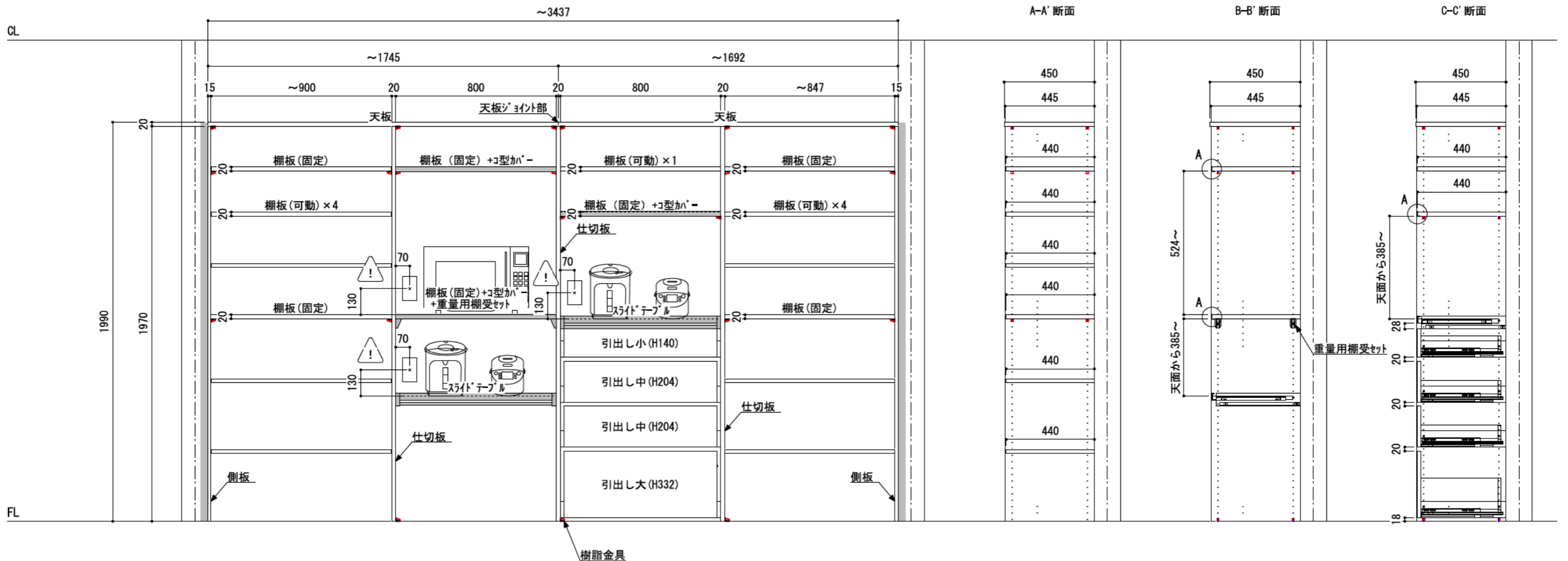
A-詳細図
